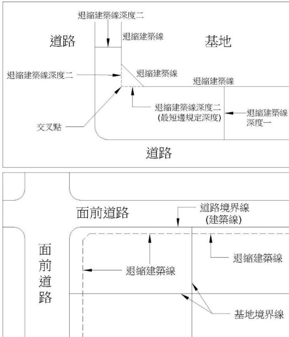
圖 1 臨計畫道路之退縮建築線示意圖
